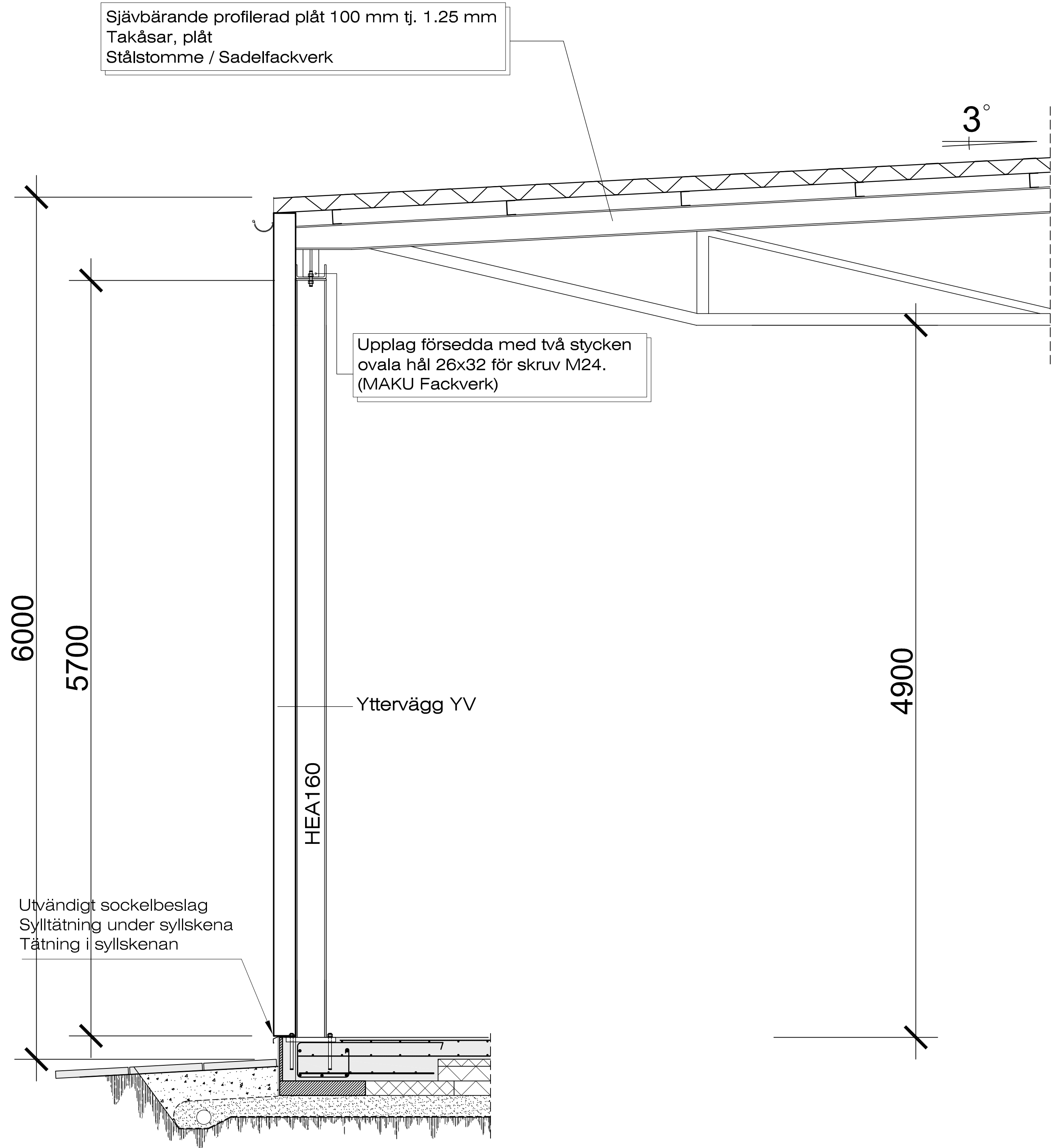
Sektion A-A skala1:20
